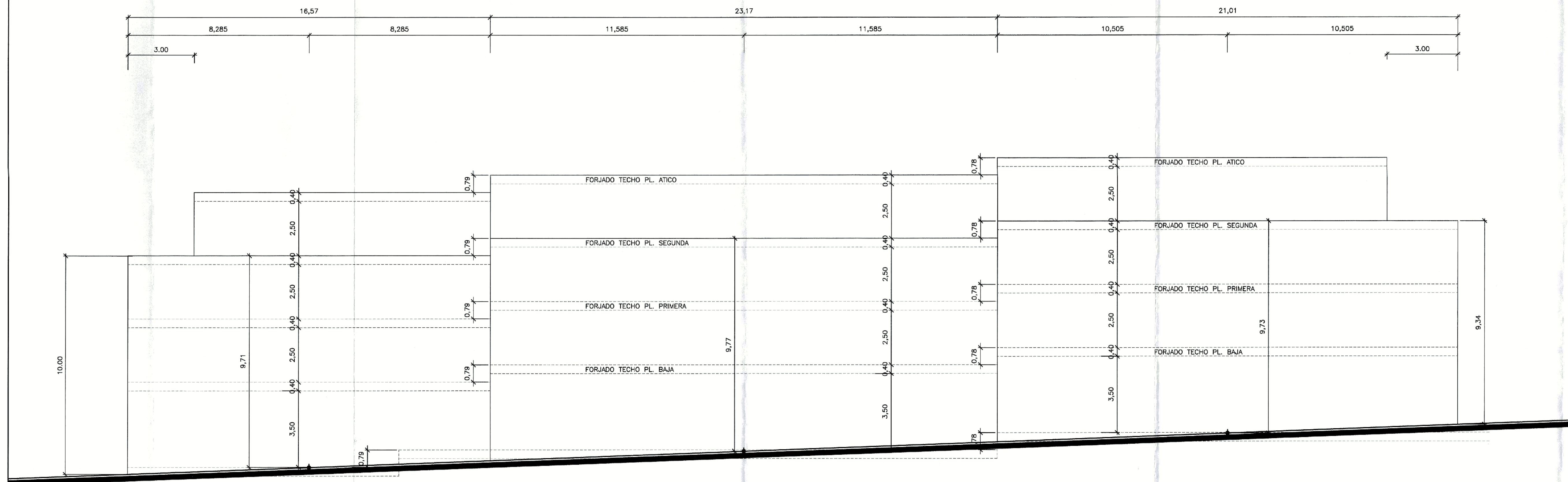
ALZADO POSTERIOR
