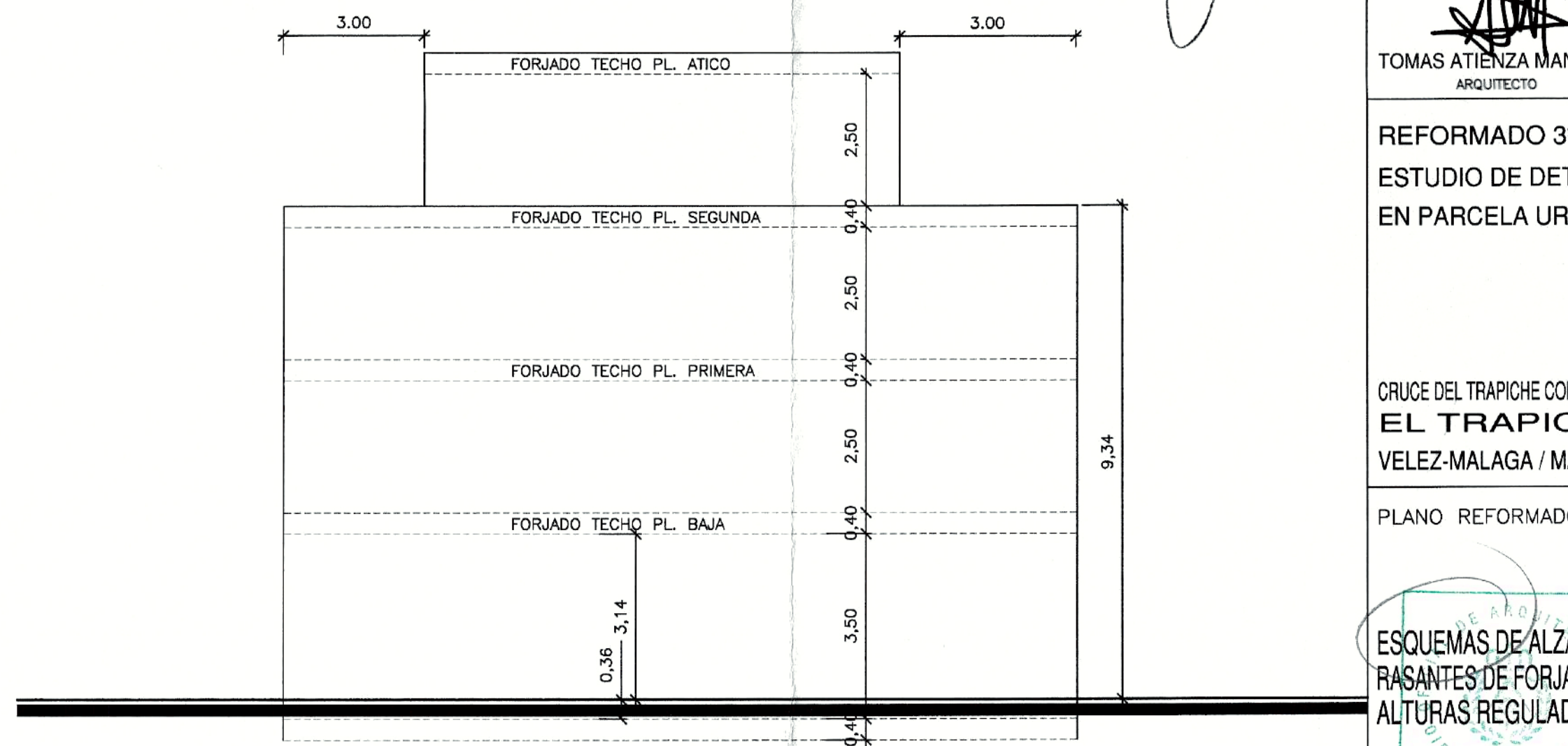
ALZADO LATERAL IZQUIERDO
