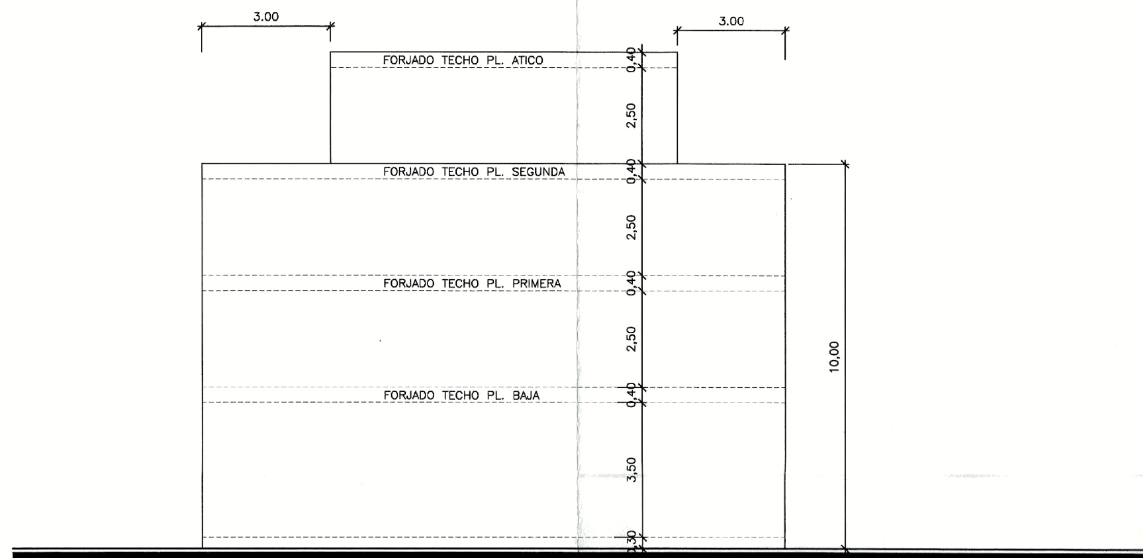
ALZADO LATERAL DERECHO
